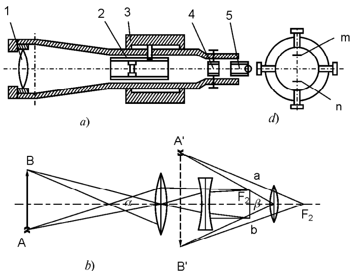
35- rasm. Ichki fokuslanuvchi ko‘rish trubasi: a — trubaning tuzilishi; b — ko‘rish trubasida nurlarning yo‘li; d — to‘rli diafragma.
