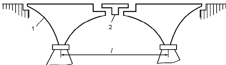
193- rasm. Balkali konsolli. 1 — konsol; 2 — osma blok.
