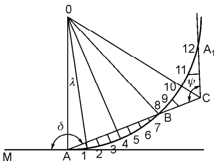
118- rasm. Kesuvchi chiziq usuli.
