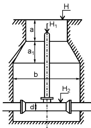
164-rasm. Vodoprovod qudug'ining tiklik qirgimi.
