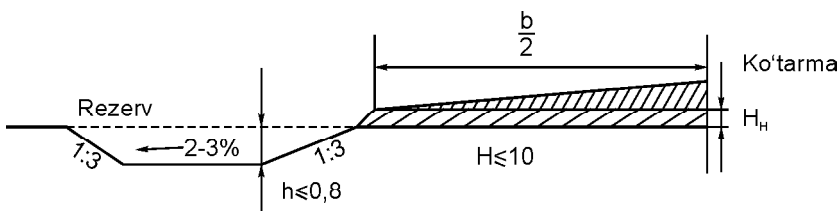
132- rasm. Yo'lining ko'tarmadagi ko'ndalang qirqimi yarmi.
