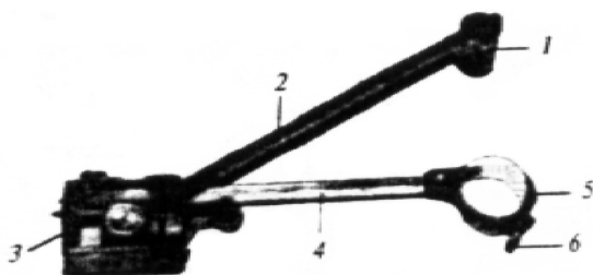
92- rasm. ПП—М qutbli planimetr: 1 — qutb; 2 — qutbli richag; 3 — sanoq olish mexanizmi; 4 — aylanish richagi; 5 — aylantirish indeksi; 6 — dasta.
