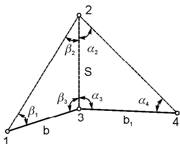
41- rasm. Bevosita o'lchab bo'lmaydigan masofani aniqlash.
