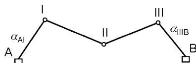
96- rasm. Taxeometrik yo'l sxemasi.
