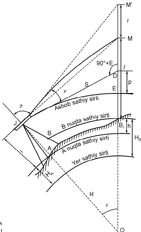
95- rasm. Nis nivelir
