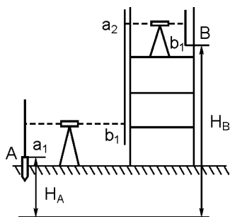
109- rasm. Balandlikni inshoot yuqori qismiga uzatish sxemasi.
