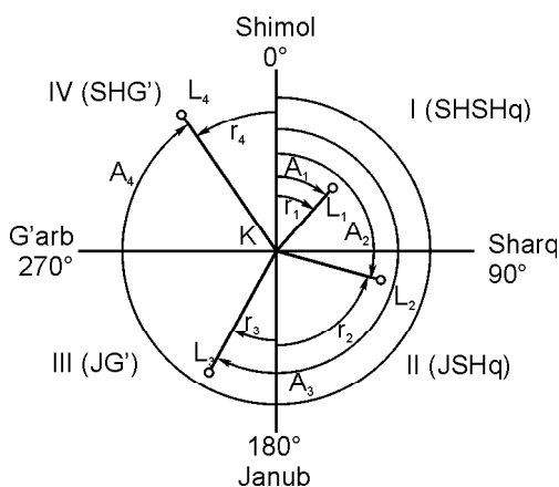
16- rasm. Chiziqlar azimutlari va rumblari orasidagi bog'lanish.
