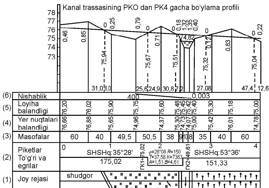
59- rasm. Kanal trassasining bo'ylama va ko'ndalang profilari.
