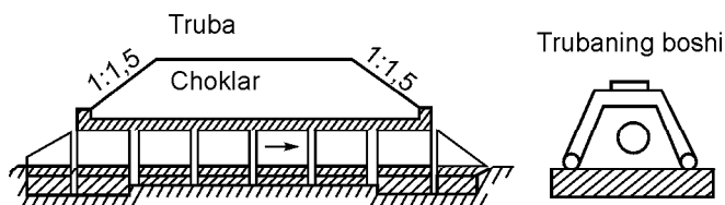
185- rasm. Bo'ylama qirgim. Ko'ndalang qirgim.
