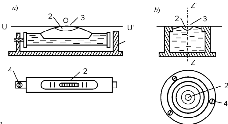
34- rasmda a) silindrik, b) doiraviy geodezik asboblardagi adilaklar.
