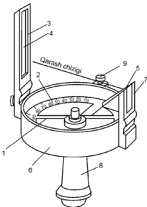
17- rasm. Dioptrlı bussol: 1 — bussol mili; 2 — gradusli halqa; 3 — narsa dioptri; 4 — ip; 5 — ko‘z dioptri; 6 — korpus; 7 — tor yoriq; 8 — dasta; 9 — mahkamlash vinti.
