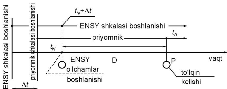
74- rasm. Psevdouzoqlikni o'lchash prinsipi.
