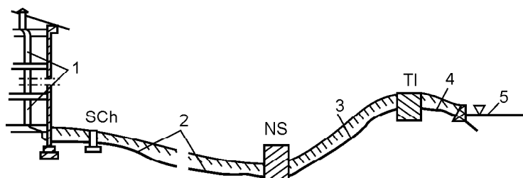
154-rasm. Kanalizatsiya tarmog'i va inshootning sxemasi.
