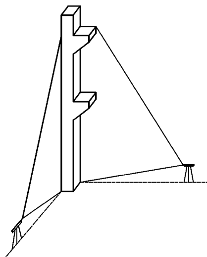
o'rnatilayotganligini lazer teodoliti yordamida aniqlash.
