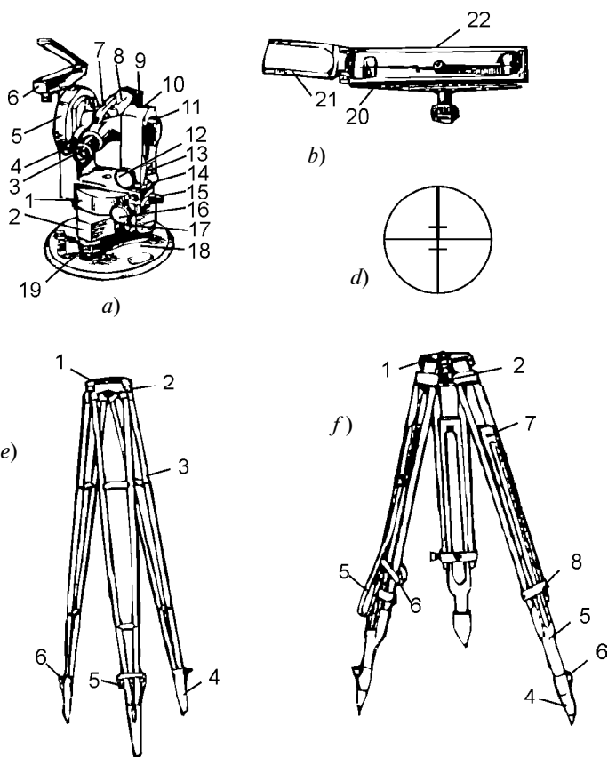
32- rasm. 3T30Π teodoliti (a), oriyentirlash bussoli (b), trubaning koʻrish maydoni (d):
