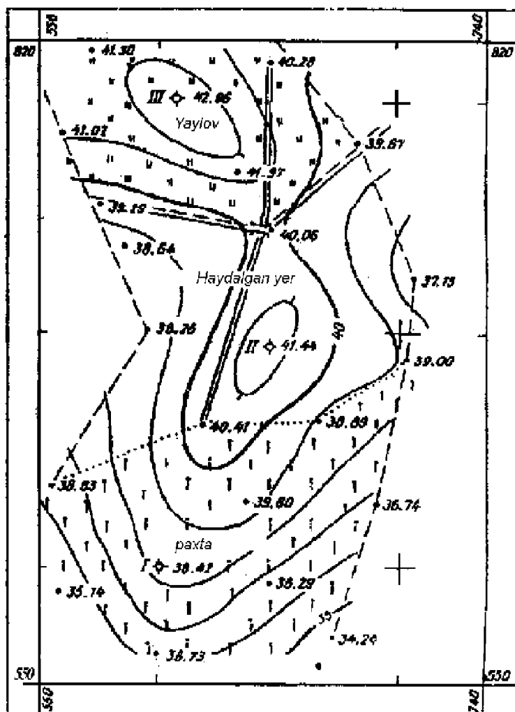
98- rasm. Taxeometrik syomka 2002, 1:1000. Relyef kesimi balandligi 1 m.
