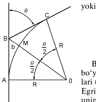
110- rasm. Burilish elementlari.
