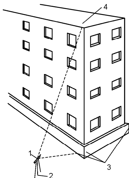
177- rasm. Bino o‘qini binoning baland qavatiga teodolit yordamida tarhlab uzatish sxemasi.
