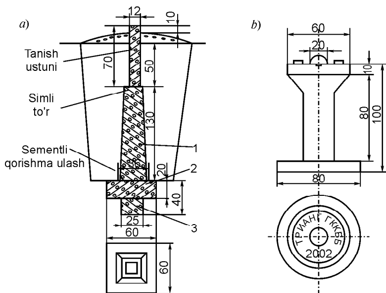
68- rasm. Belgilar markazlari: a — punkt markazi; b — cho'yan marka.
