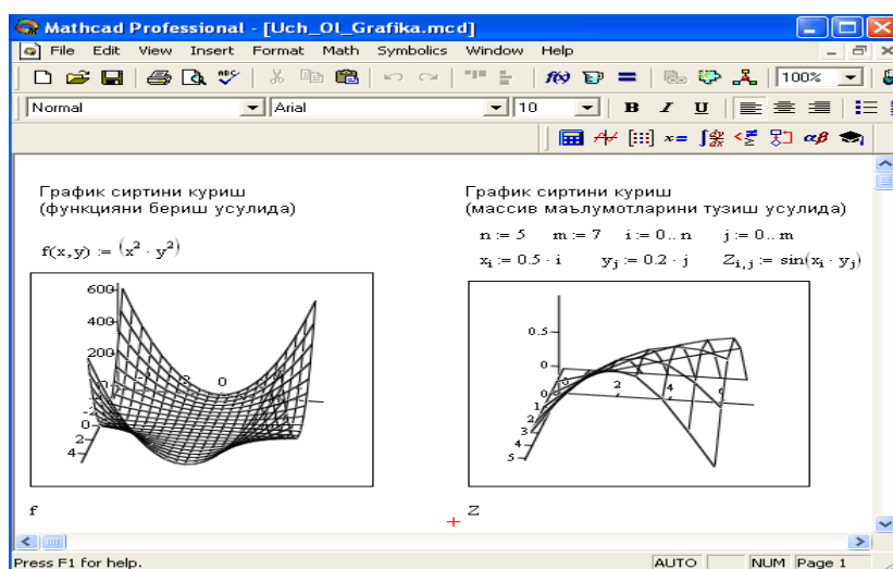
5-rasm. Uch o'zgaruvchili funktsiya grafigini qurish
