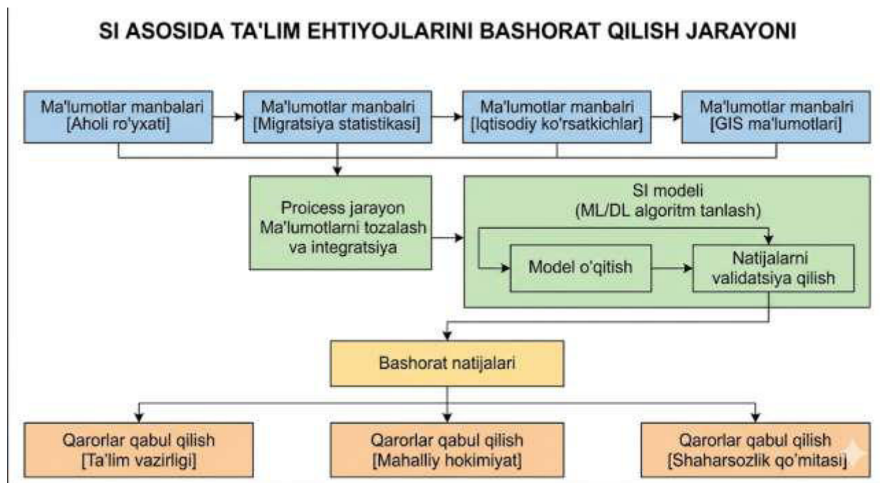
2-rasm. SI asosida ta'lim ehtiyojlarini bashorat qilish jarayonining blok-sxemasini
