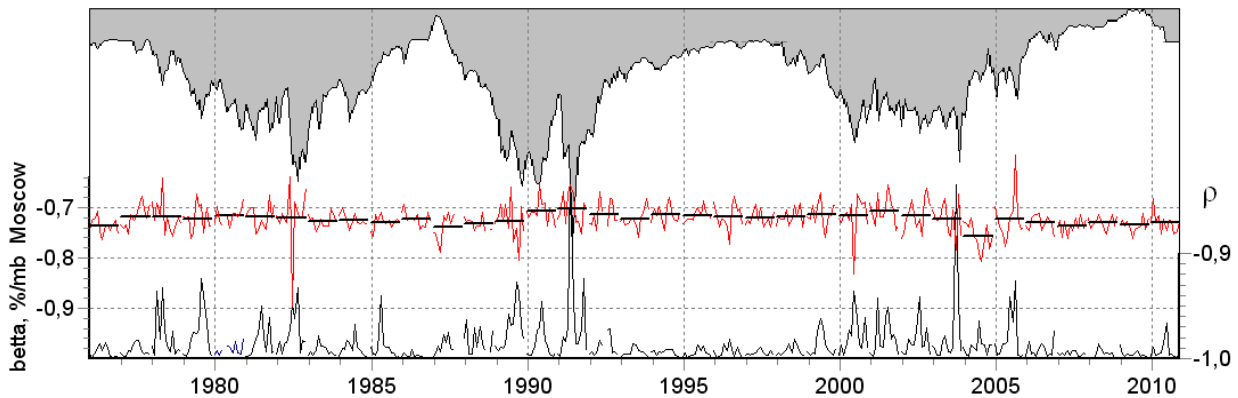
Рис. 6. Результат анализа барометрического эффекта станции Москва, исправленная на вариации по данным станции Newark
