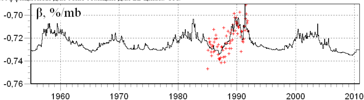
Рис.10. Среднемесячные значения барометрического коэффициента для nm64 Москва за весь период наблюдений
