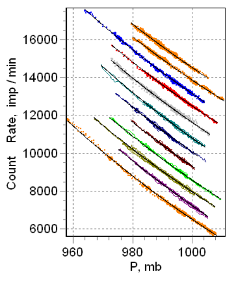
Рис 3. Зависимость скорости счета детектора от атмосферного давления для 2009 года для спокойного периода
