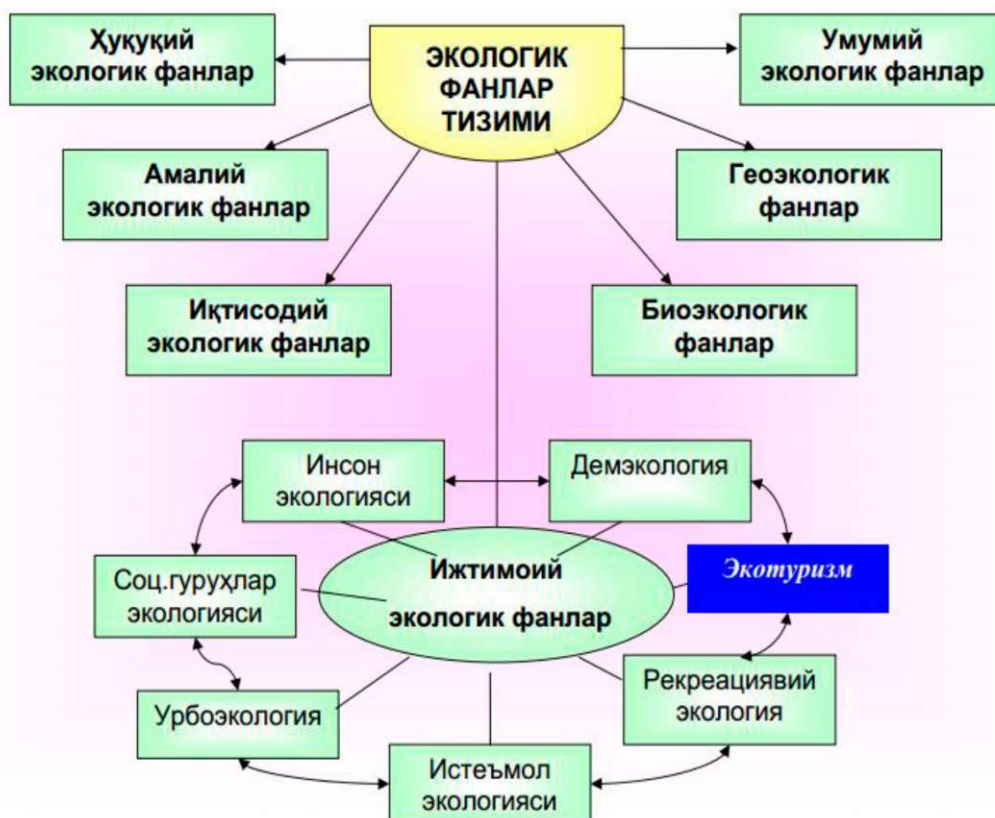
1-чизма. Экотуризмнинг экологик фанлар билан боғланганлиги
