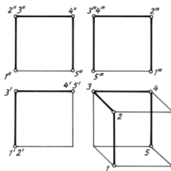
1-rasm. Simdan yasalgan modelning ko'rinishlari.
