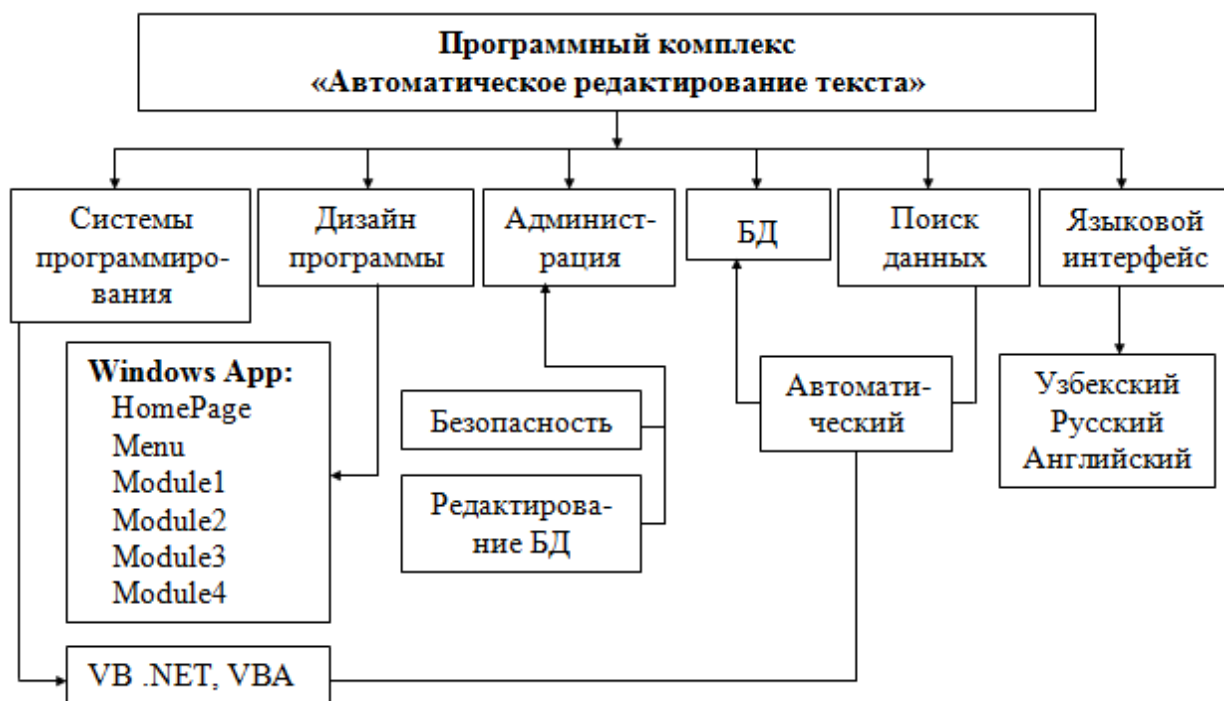
Рис. 1. Архитектура программного комплекса «Автоматическое редактирование текста»
