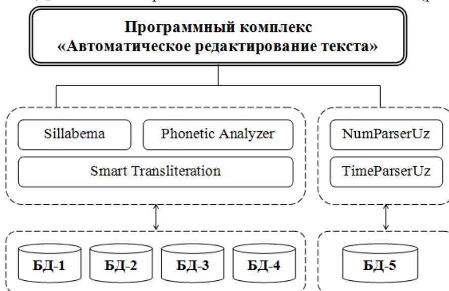
Рис. 3. Интеграция программного комплекса с БД
