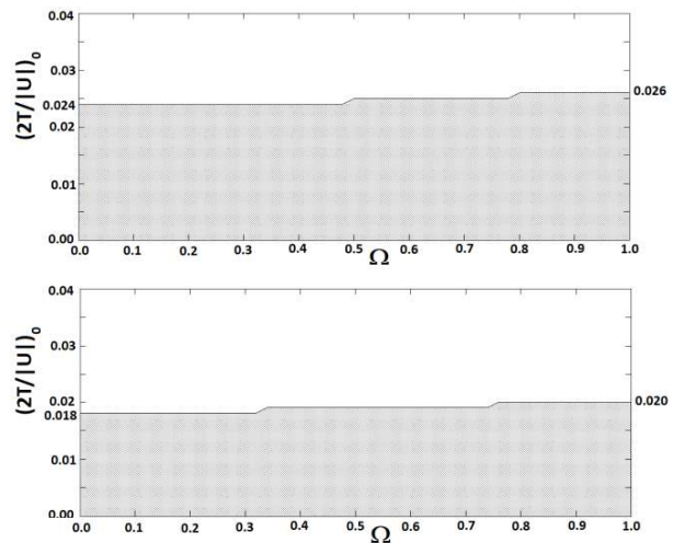
Рис. 1. Критические зависимости начального вириального отношения от параметра вращения (вверху для N=14 , m=5 и внизу для N=16 , m=6 ). Неустойчивости от (2T/|U|)_0 и \Omega (вверху для N=14 , m=5 и внизу для N=16 , m=6 ). Цифрами у кривых обозначены значения параметра вращения.
