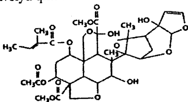
Azadiraxtin
