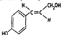
Para-kumar spirti
