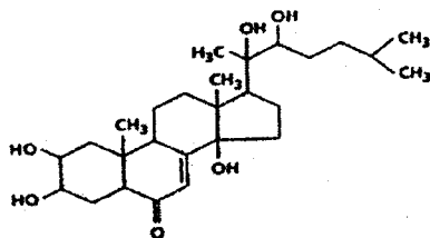
Ponasteron A
