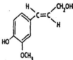
Koneferil
