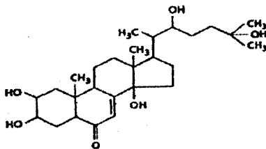
\alpha - Ekdizon
