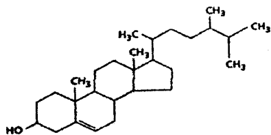
Sitosterol
