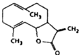
Kostunolid
