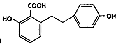
Lunular kislotasi
